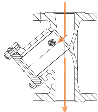
Einbaulage vertikal
