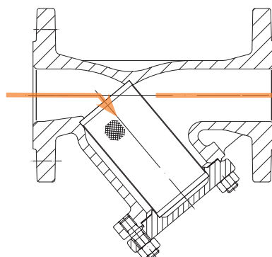
Einbaulage horizontal
